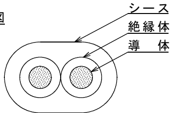
構造図
